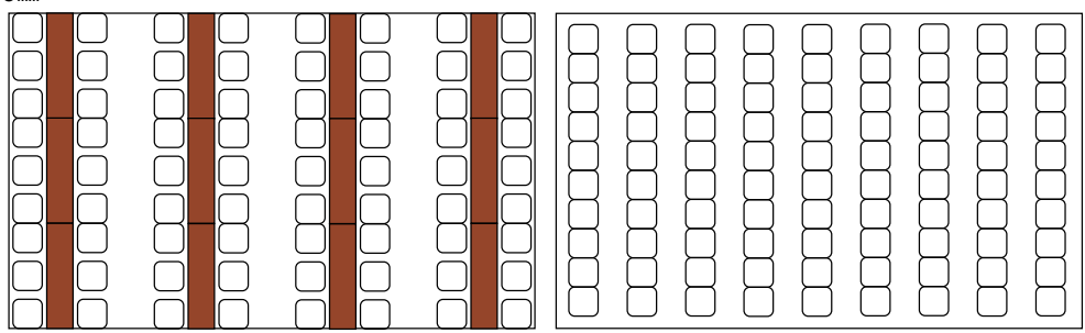
■3k x 6k テント寸法図面 8本柱
