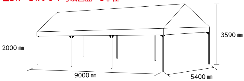
■3k x 5k テント寸法図面 8本柱
