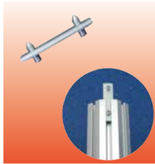
■コネクタプレート サイズ：W40×H10mm 重量：0.008kg ※止めネジM4×12mm2本付 ※10mmミゾの深さ用
