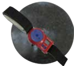
■ジャンプメーター サイズ: W137×D35×H80mm ゴム板: 直径380mm 厚さ3mm 測定範囲: ベルト高さ110cmで5~99cm 重量: 0.2kg (ゴム板0.4kg) 電源: リチウム電池内蔵
