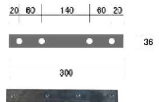
■フラットバー（スチール） サイズ：W300×D36×H3mm ※両面パネルの連結で使用します パネルの上下に設置してビスで固定します。
