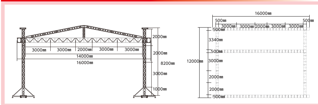
■ ルーフトラスシステム16×12m図面
