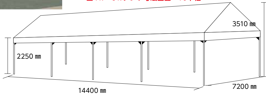
■4k×8kテント寸法図面 10本柱
