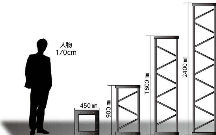
■黒アルミトラス (450mm)
