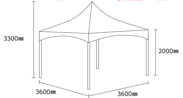
■2k×2kテント寸法図面 4本柱
