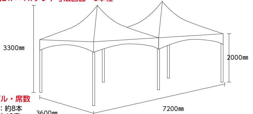
■2k×4kテント寸法図面 6本柱
