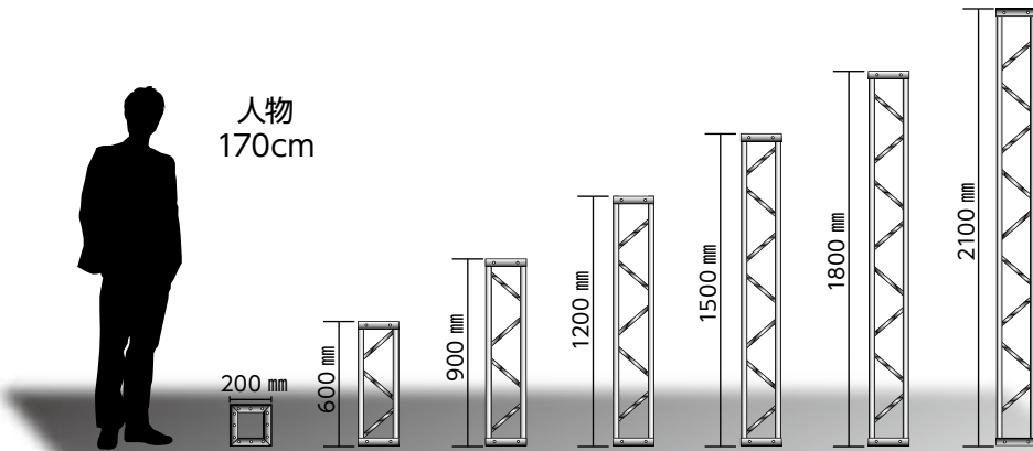
■アルミトラス (200mm)
