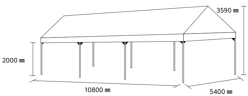
■3k x 6k テント寸法図面 8本柱
