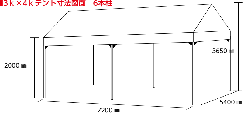
■3k x 4k テント寸法図面 6本柱
