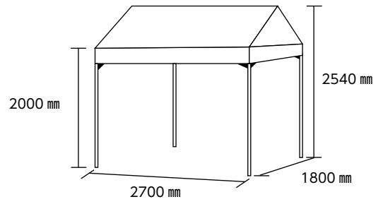
■1k×1.5kテント寸法図面 4本柱
