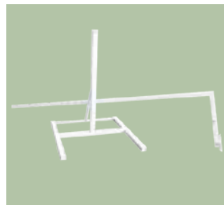
■くす玉スタンド 合計サイズ: H3860×D1110×W800mm 上部サイズ: H2550×D710×W350mm 下部サイズ: H1310×W800×D850mm
