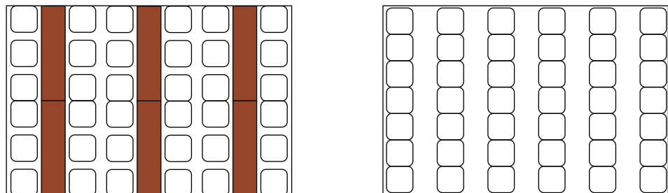
■1.5k x 2k テント寸法図面 4本柱
