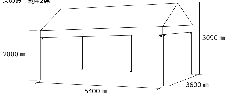
■5本足 2k×3kテント寸法図面
