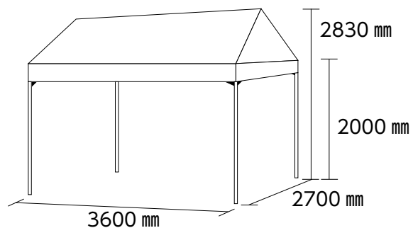
■1.5k x 2k テント寸法図面 4本柱
