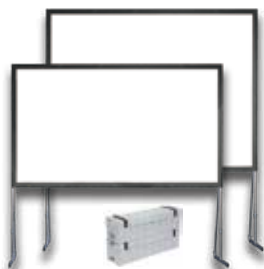
■303インチ(組立式 16:9) スクリーンサイズ: W6910×H3970mm イメージサイズ: W6710×H3770mm サイズ: W6910×H4157~5987×D1131mm 重量: 61kg
