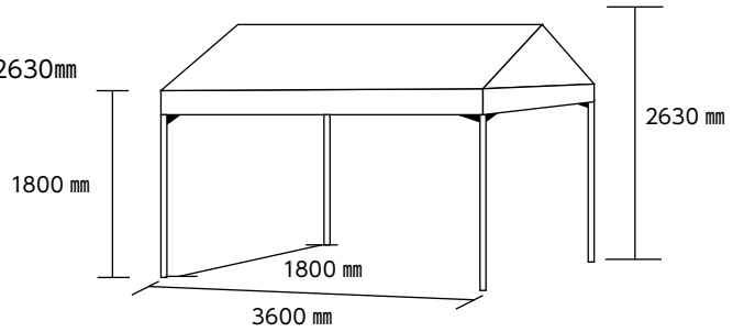
■1k×2kテント寸法図面 4本柱
