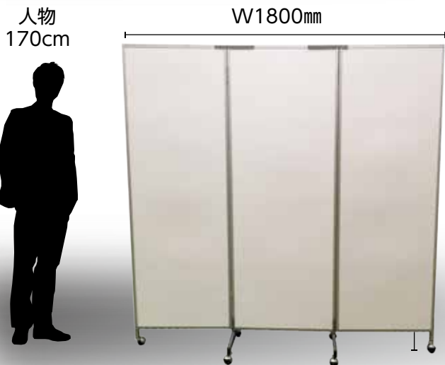
■三つ折パーテーション サイズ：W1800×H1800mm (足H120mm含) 両端パネル：W585 × H1800mm (足120mm含) 中央パネル：W624 × H1800mm (足120mm含)
