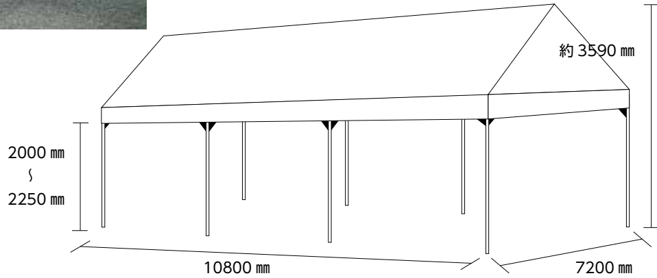
■4k×6kテント寸法図面 8本柱
