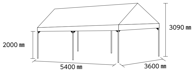
■2k x 3k テント寸法図面 6本柱
